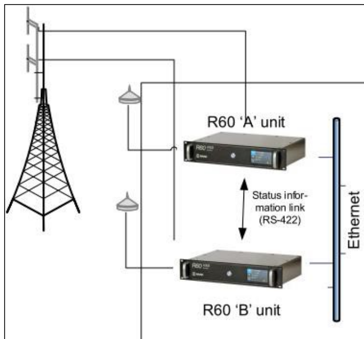
Figura 4-1 Configuración de espera activa
